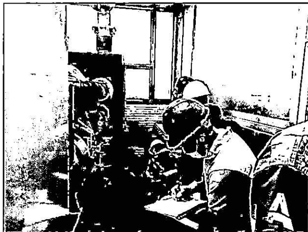
Medición de flujo de gases de cárter del motor 3406
