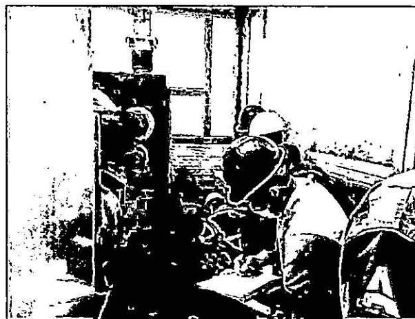
Medición de flujo de gases de cárter del motor 3406
