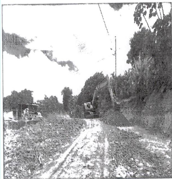
Fotografía 6.- Ampliación de la mesa vial
