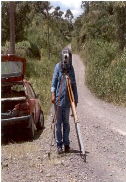
OPERANDO ESTACION TOTAL
